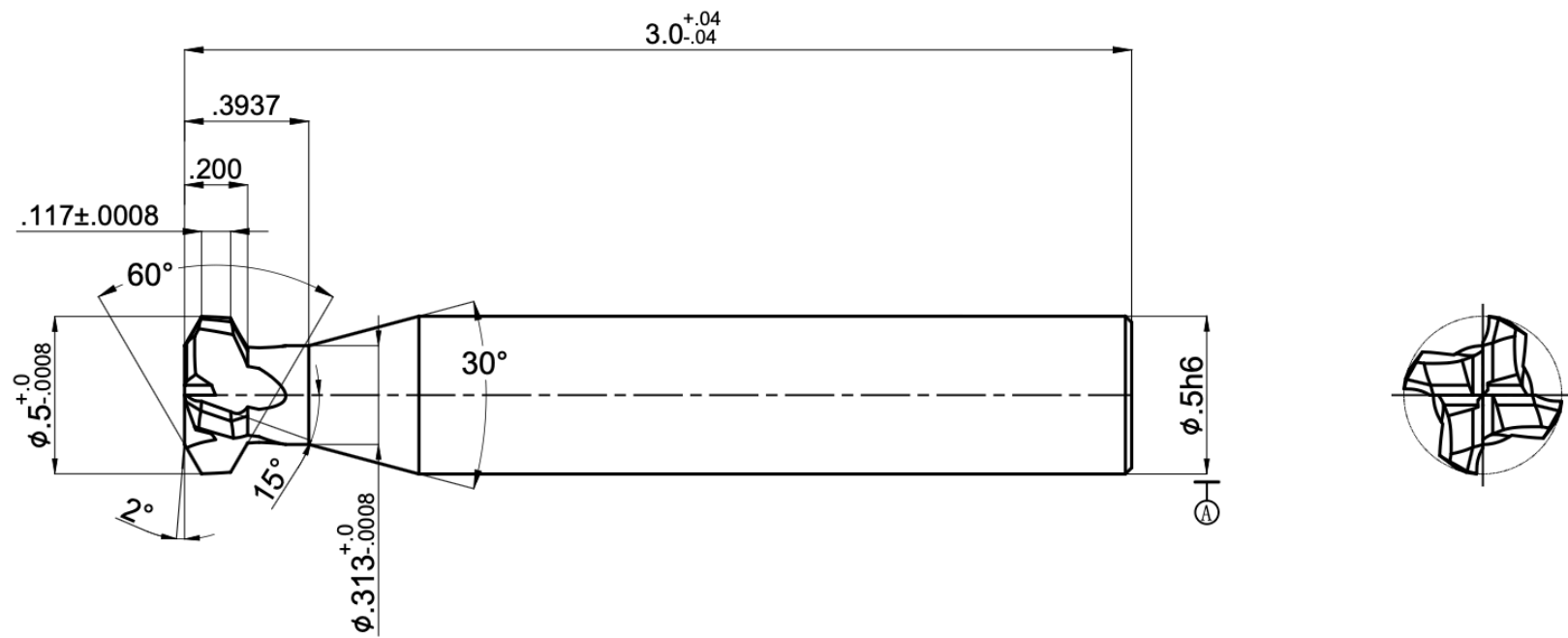
Maritool Part# 1311SP-.500-1
